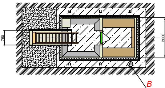
Разрез Б-Б
