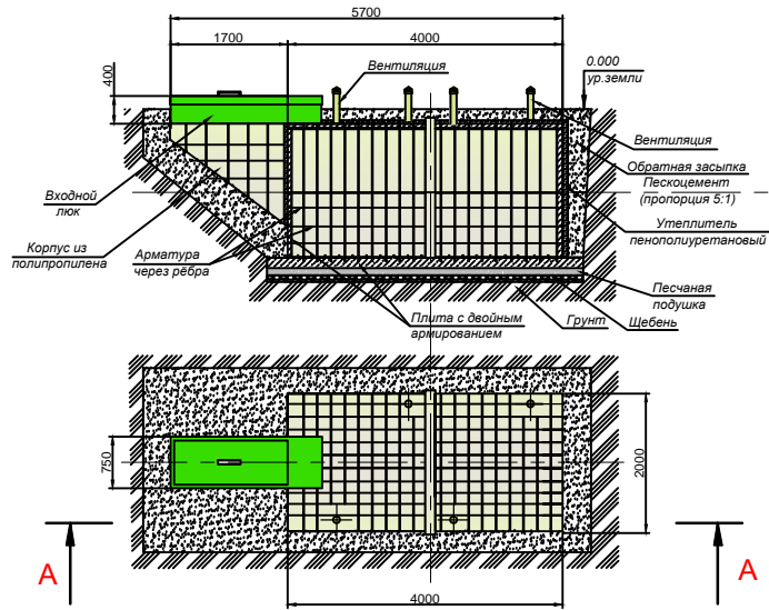
Разрез А-А
