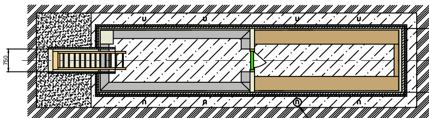
Разрез Б-Б
