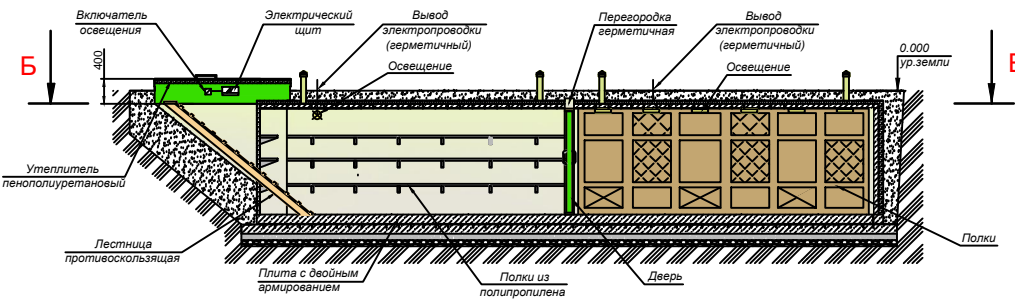
Разрез Б-Б
