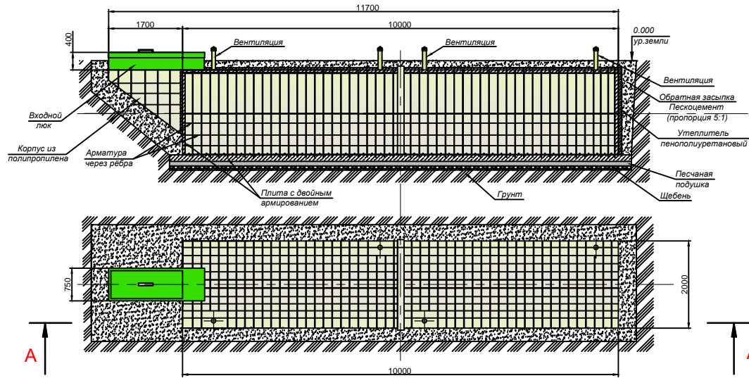
Разрез А-А
