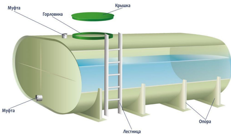
Рисунок 8. ГРИНЛОС Емкость горизонтальная овальная наземная в разрезе
