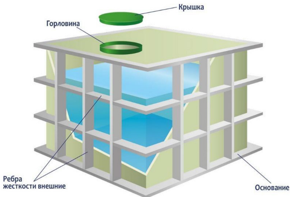
Рисунок 10. ГРИНЛОС Емкость прямоугольная наземная в металлическом каркасе в разрезе
