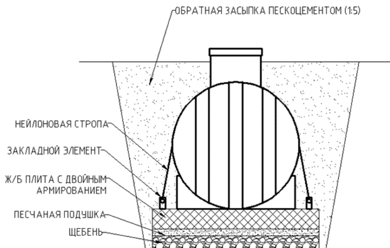
Схема 2. Установка Изделия в котлован
