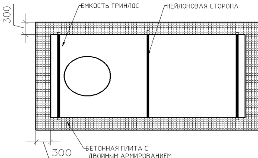
Схема 1. Котлован вид сверху
