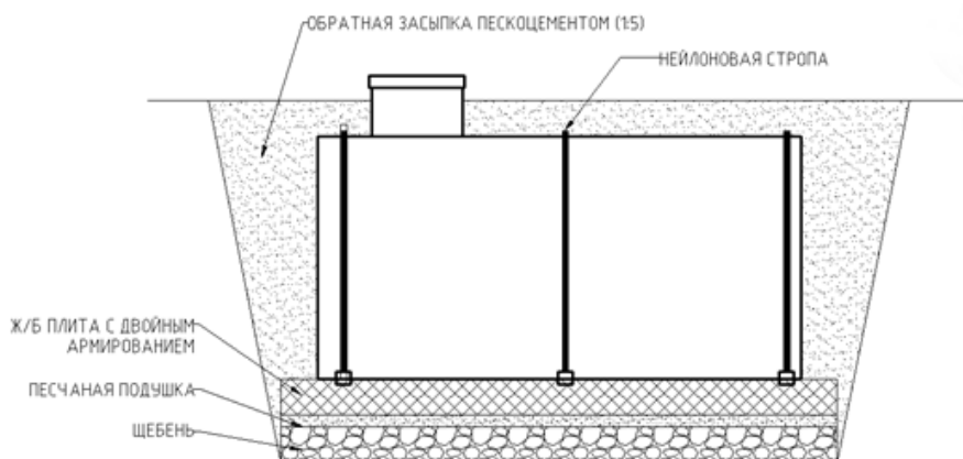
Схема 3. Установка Изделия в котлован вид сбоку
