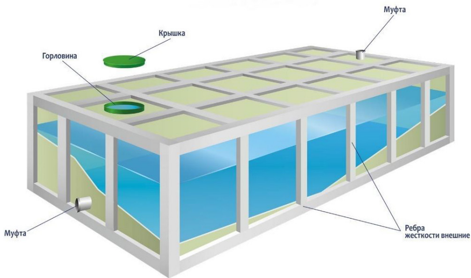
Рисунок 12. ГРИНЛОС Емкость прямоугольная наземная в металлическом каркасе в разрезе
