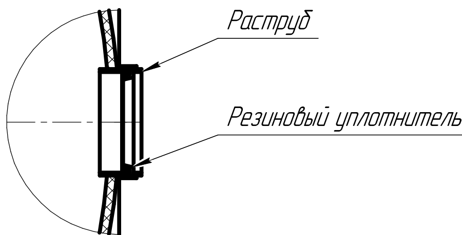
А(1:4) 2 места
