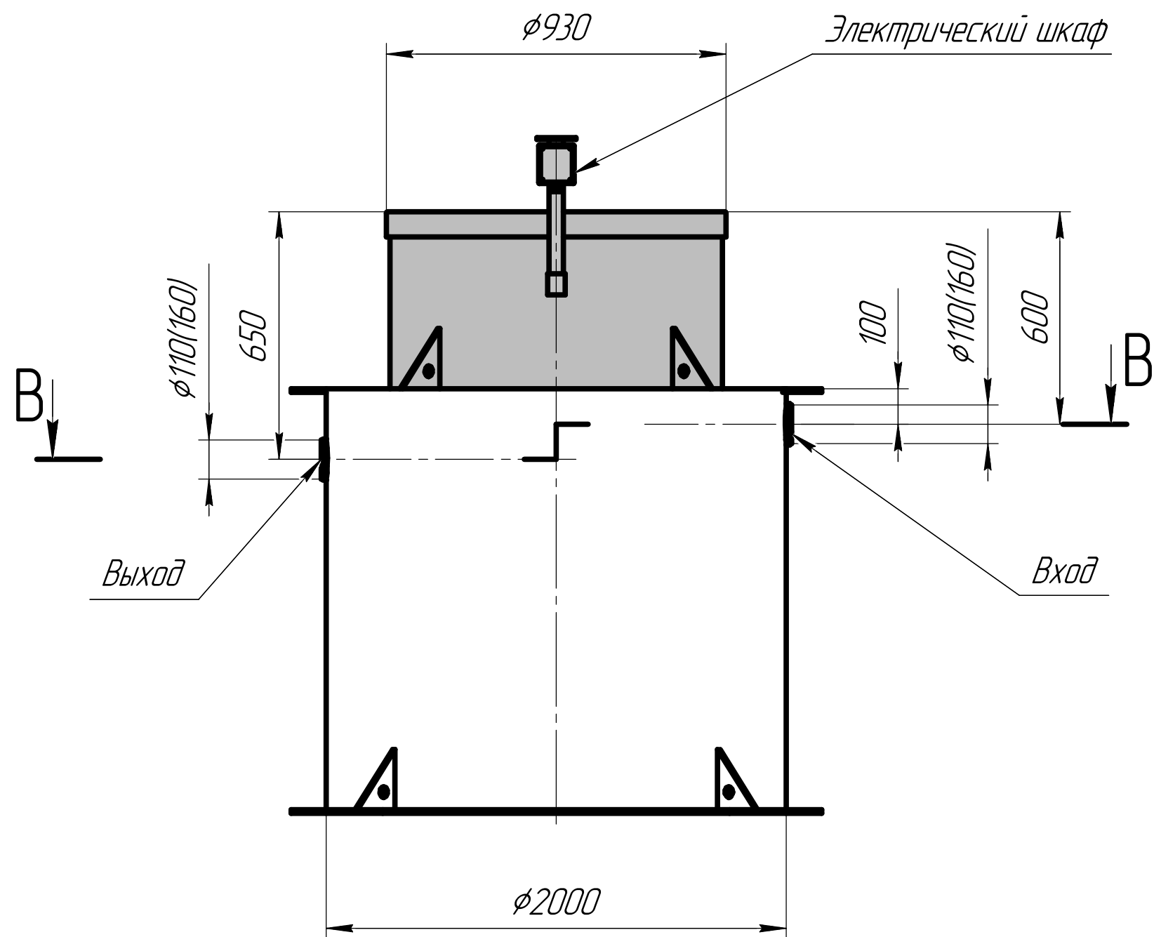
Вид спереди
