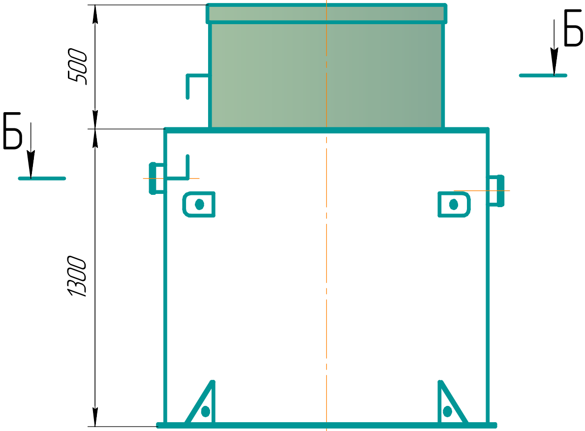
Вид спереди
